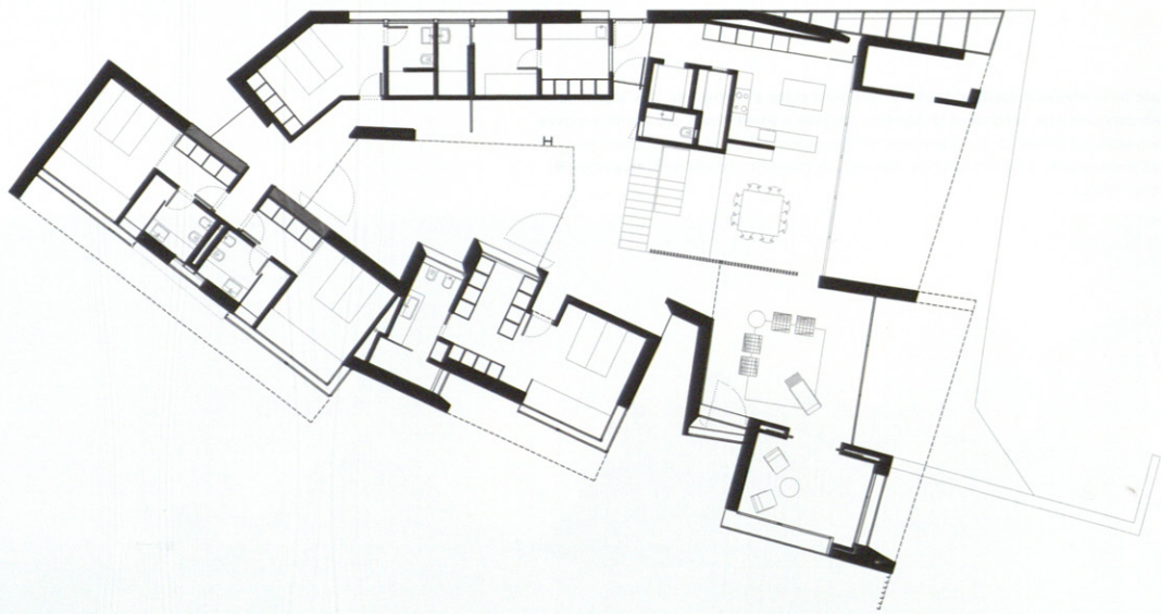
PLANTA BAJA. GROUND FLOOR.
